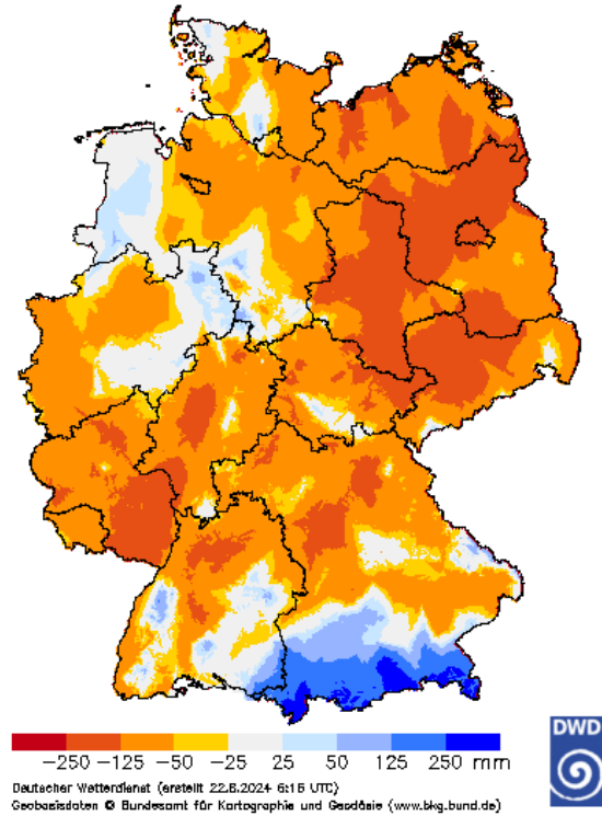
Klimatische Wasserbilanz mit Grasreferenzverdunstung 01.06.2024–21.08.2024
