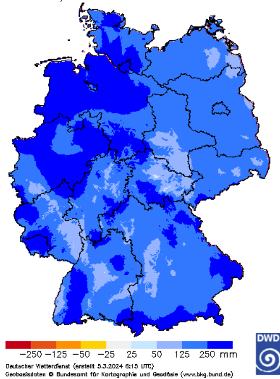
Klimatische Wasserbilanz mit Grasreferenzverdunstung Winter 2023/2024
